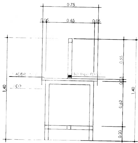
VISTA 02 S/ESCALA
