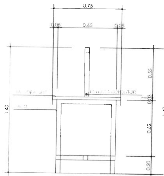
VISTA 04 S/ESCALA
