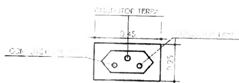
DETALHE - TOMADA FÊMEA S/ESCALA
