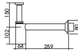
1680 C 112** sifão para cozinha/tanque
