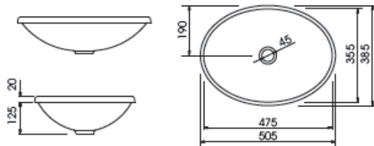
Cuba de sobrepor oval DECA L.680 na cor branco ou equivalente técnico.
