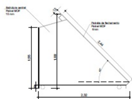
VISTA LATERAL ESQUERDA ESC.: 1/25
