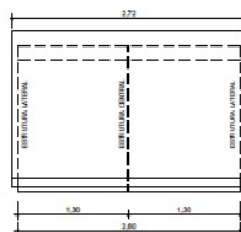
VISTA FRONTAL ESC.: 1/25
