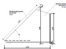
VISTA LATERAL DIREITA ESC.: 1/25
